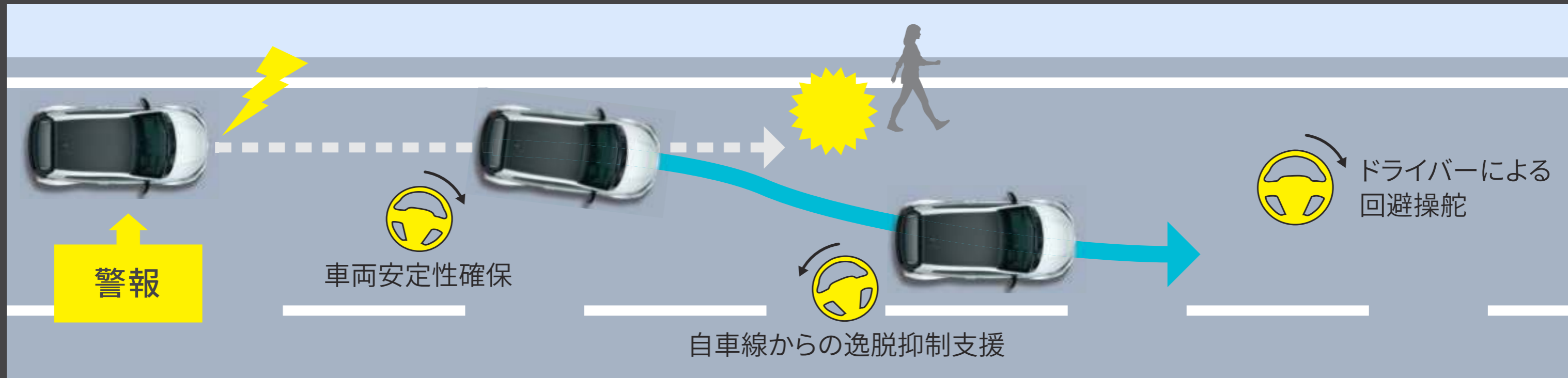
緊急時操舵支援機能の作動イメージ [自車線内の歩行者との衝突回避操作を支援]
